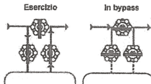
Sistema di By-pass classico
